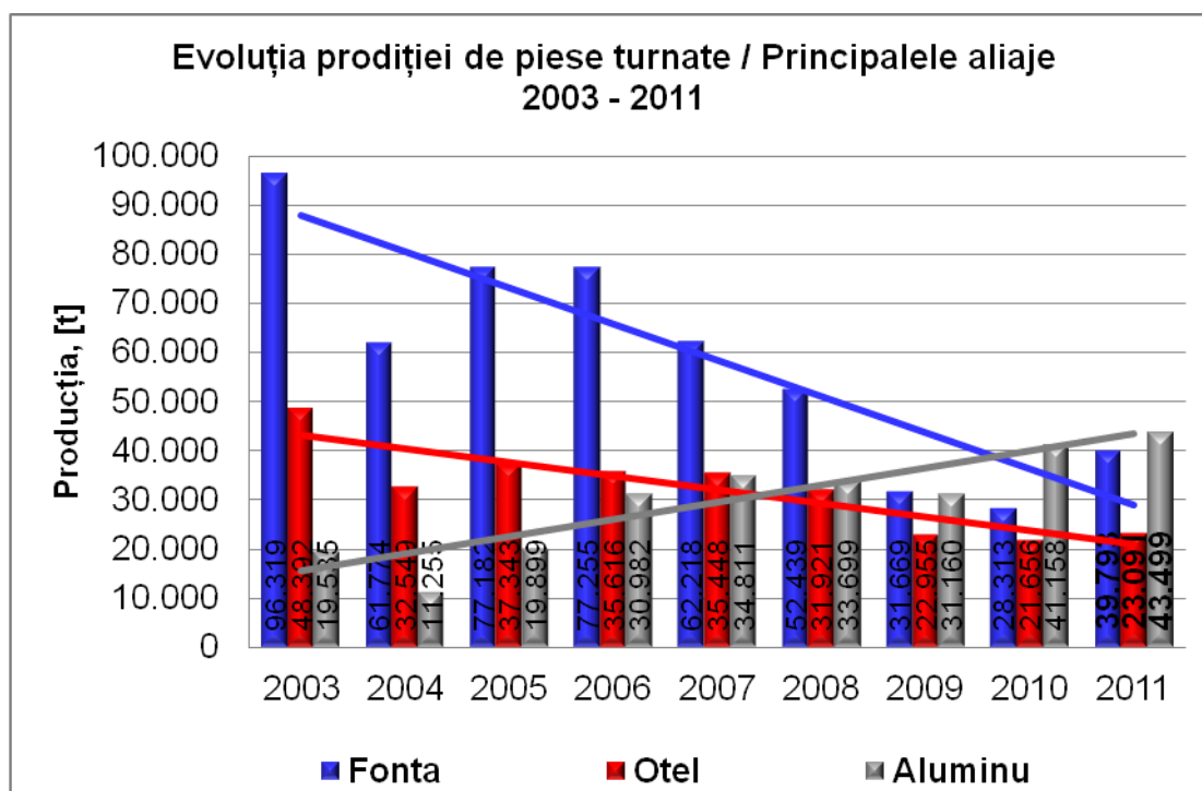
Figura 3. Evoluția produției de piese turnate, principalele aliaje, 2003 – 2011
