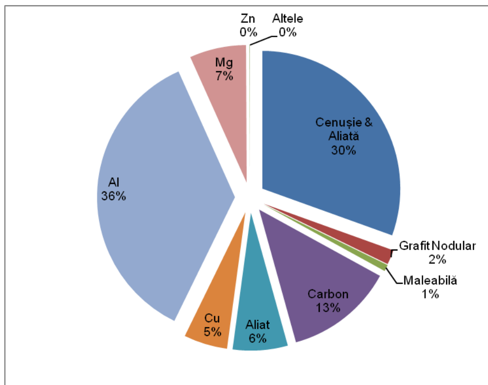
Figura 3. Repartiția cantitativă a principalelor aliaje de turnătorie, în producția anului 2011
