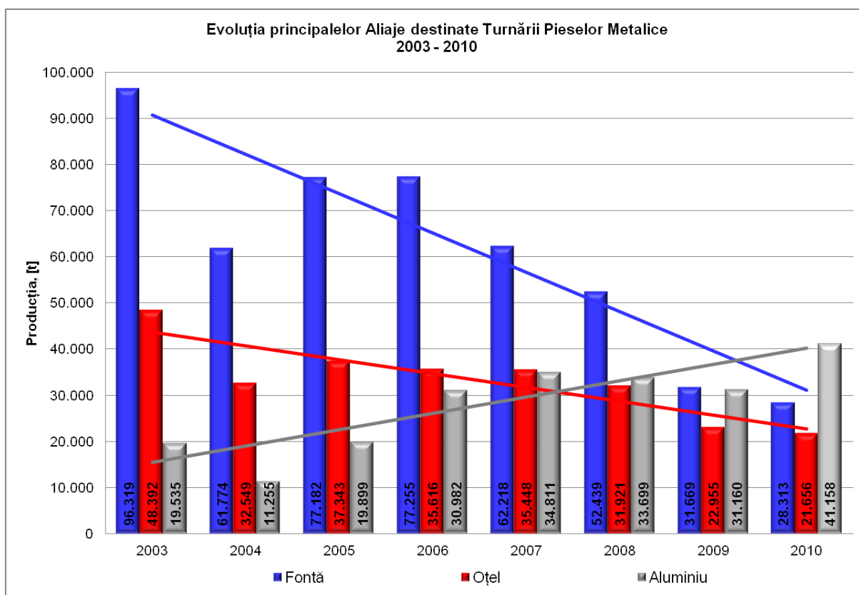
Figura 3. Evoluția producției de piese turnate, principalele aliaje, 2003 - 2010
